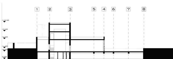
SECȚIUNE A - A' SC 1 : 200
